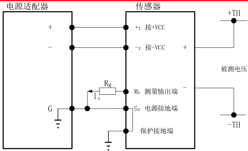
图 3 电气连接图
