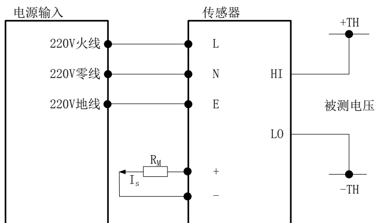
图 3 电气连接图
