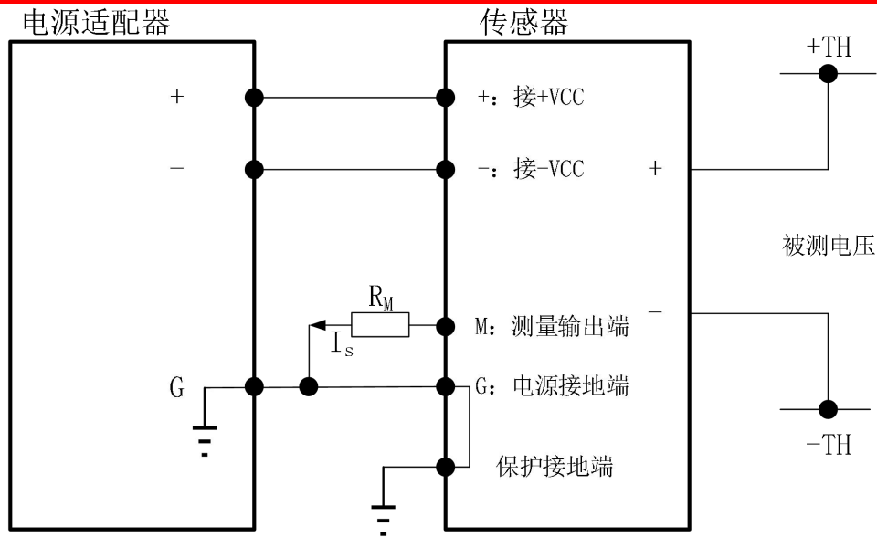
图 3 电气连接图
