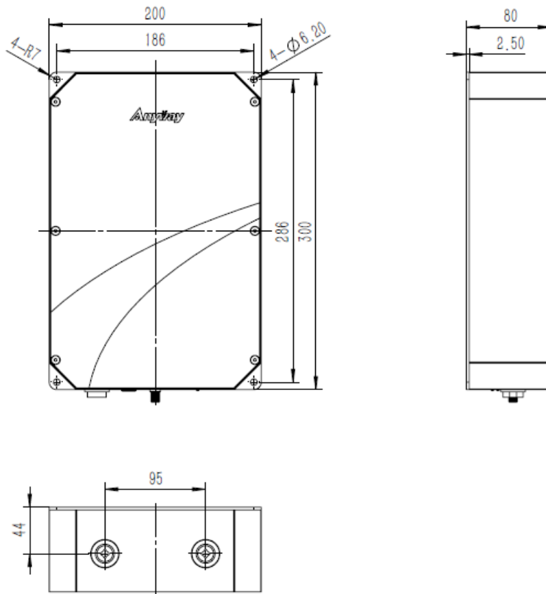
图 1 外形图
